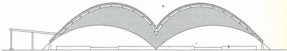
Fachada com anteparo do Galpão da Fazenda Tecelagem Parahyba em São José dos Campos
