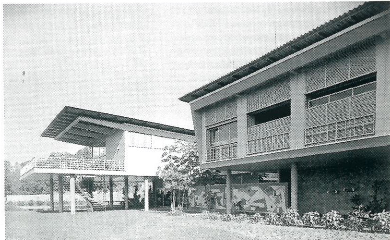
Residência Olivo Gomes, atual Parque da Cidade, S. J. Campos. Foto Acervo Digital Rino Levi FAU PUC-Campinas
